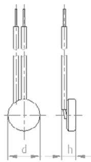
Bauhöhe h ab 3,9 mm Durchmesser d 9,0 mm
